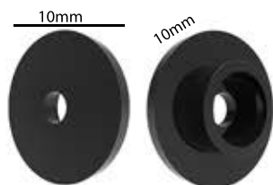
Ref.: APBP 001 MACHO Espessura: 2,7mm Materiais: POM Embalagem: 1000 unidades
