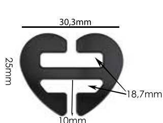
Ref.: APJ 003 10mm Espessura: 1,7mm Materiais: POM e PC Embalagem: 100 unidades
