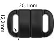
Ref.: APF 002 8mm Espessura: 3,6mm Materiais: POM, PC e HS Embalagem: 500 unidades
