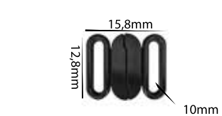
Ref.: APF 019 10mm Espessura: 2,5mm Materiais: POM, PC e HS Embalagem: 1000 unidades
