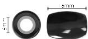
Ref.: APPON 001 16x6mm Espessura: 2,3mm Materiais: POM e PS Embalagem: 100 unidades
