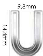
Ref.: AML U Passante interno: 12mm Material: zamac Espessura: 4,5mm
