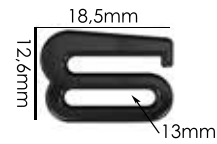
Ref.: APG 001 13mm Espessura: 1,7mm Materiais: POM, PC e HS Embalagem: 1000 unidades
