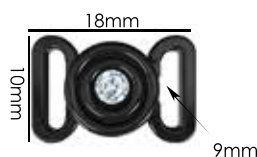
Ref.: APF 002 8 e 10mm Espessura: 2,8MM Materiais: POM e PC Acabamentos: Cristal ou Oktant Swarovski Embalagem: 100 unidades
