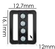
Ref.: APR 004 12mm Espessura: 2,1-mm Materiais: POM, PC e HS Acabamentos: Cristal ou Oktant Swarovski Embalagem: 100 unidades
