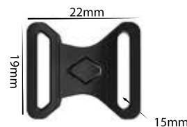
Ref.: APF 026 15mm Espessura: 2,4mm Materiais: POM, PC e HS Embalagem: 1000 unidades
