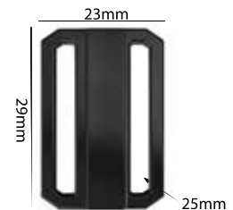
Ref.: APF 031 25mm Espessura: 5mm Materiais: POM e PC Embalagem: 500 unidades
