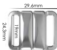
Ref.: AMF 024 19mm
