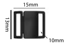
Ref.: APF 023 10mm Espessura: 3mm Materiais: POM, PC e HS Embalagem: 1000 unidades
