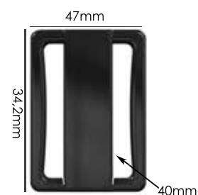
Ref.: APP 005 40mm Espessura: 3,7mm Materiais: POM, PS e HS Embalagem: 100 unidades
