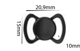
Ref.: APF 014 10mm Espessura: 2,7mm Materiais: POM, PC e HS Embalagem: 1000 unidades
