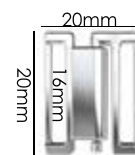
Ref.: AMF 022 16mm
