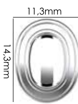
Ref.: AML O Passante interno: 12mm Material: zamac Espessura: 4,5mm
