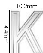
Ref.: AML K Passante interno: 12mm Material: zamac Espessura: 4,5mm
