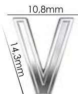
Ref.: AML V Passante interno: 12mm Material: zamac Espessura: 4,5mm
