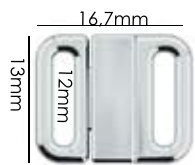
Ref.: AMF 017 12mm
