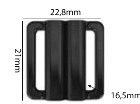
Ref.: APF 010 16,5mm Espessura: 3,8mm Materiais: POM, PC e HS Embalagem: 200 unidades
