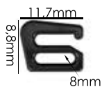
Ref.: APG 000/B 8mm Espessura: 1,3mm Materiais: POM, PP, PC e HS Embalagem: 1000 unidades
