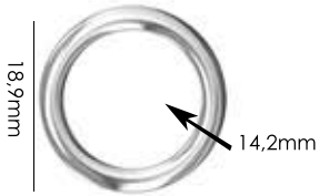
Ref.: AMA 014 14,2mm Material: zamac
