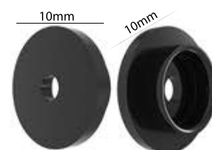
Ref.: APBP 001 FÊMEA Espessura: 2,7mm Materiais: POM Embalagem: 1000 unidades
