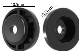
Ref.: APBP 003 FÊMEA Espessura: 3mm Materiais: POM Embalagem: 1000 unidades
