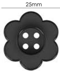
Ref.: APB 001 25mm Espessura: 2mm Materiais: POM, PC e HS Embalagem: 100 unidades
