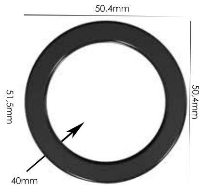
Ref.: APA PARALELA 40mm Espessura: 2,4mm Materiais: POM, PC e HS Embalagem: 200 unidades
