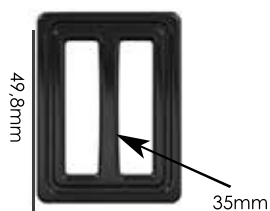
Ref.: APP 006 35mm Espessura: 3,7mm Materiais: POM, PS e HS Embalagem: 100 unidades
