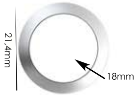
Ref.: AEA 18mm Material: aço estampado
