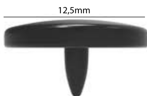
Ref.: ACABAMENTO 003 Espessura: 5mm Materiais: POM Embalagem: 1000 unidades OBS.: Pode ser vendido em conjunto com APBP 003 MC e FM
