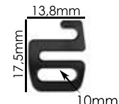
Ref.: APG 005 10mm Espessura: 2,7mm Materiais: POM e PC Embalagem: 1000 unidades
