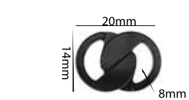
Ref.: APF 015 8mm Espessura: 2,4mm Materiais: POM, PC e HS Embalagem: 1000 unidades
