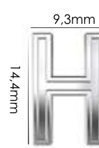
Ref.: AML H Passante interno: 12mm Material: zamac Espessura: 4,5mm
