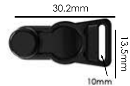
Ref.: APE 001 10mm Espessura: 1,4mm Materiais: POM e PC Embalagem: 200 unidades
