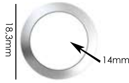
Ref.: AEA 14mm (Sob Consulta) Material: aço estampado
