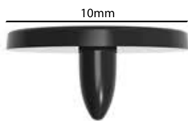
Ref.: ACABAMENTO 001 Espessura: 5mm Materiais: POM Embalagem: 1000 unidades OBS.: Pode ser vendido em conjunto com APBP 001 MC e FM
