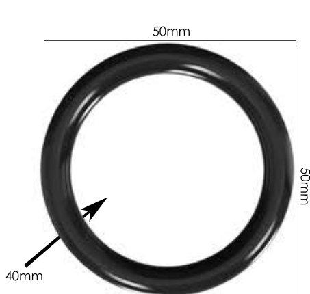
Ref.: APA 40mm/B Espessura: 5,9mm Materiais: POM, PC e HS Embalagem: 100 unidades
