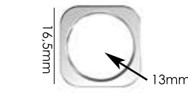
Ref.: AMA 019 13mm Material: zamac
