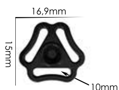
Ref.: APT 002 10mm Espessura: 2,6mm Materiais: POM e PC Embalagem: 1000 unidades
