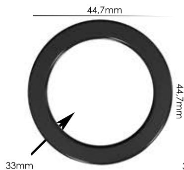
Ref.: APA PARALELA 33MM Espessura: 2,5mm Materiais: POM, PC e HS Embalagem: 200 unidades
