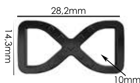
Ref.: APP 004 10mm Espessura: 2 mm Materiais: POM, PC e HS Embalagem: 1000 unidades
